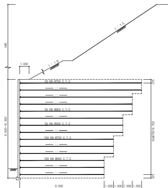
단면 M-M
